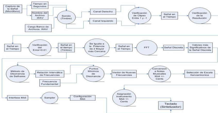
Imagen 1- Modelo Secuencial Diagrama de Flujo de Datos
